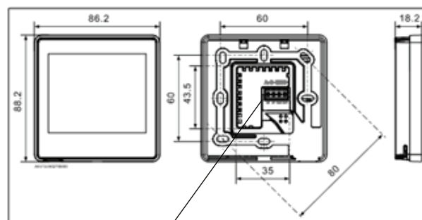
Dimensiones (mm)
