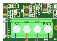
Regleta de conexionado de 3 velocidades en la PCB
