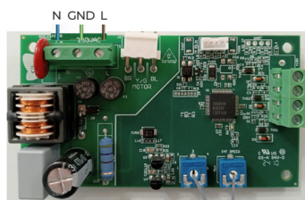
Selectores de regulación de la velocidad variable
