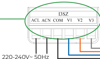
Faixa de terminal do comando
