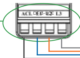
Faixa de terminal do comando
