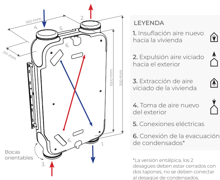
Flujos de aire versión derecha Versión de fábrica Instalación en horizontal / vertical (Instalación vertical solo con versión entálpica)
