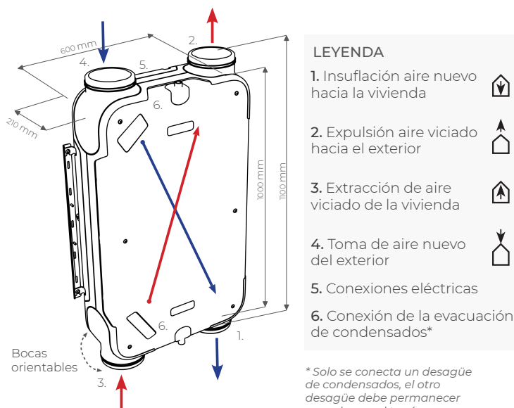
Flujos de aire versión derecha Instalación en horizontal / vertical (Instalación vertical solo con versión entálpica)
