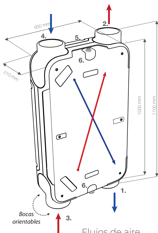
Flujos de aire Versión de fábrica Instalación horizontal en techo
