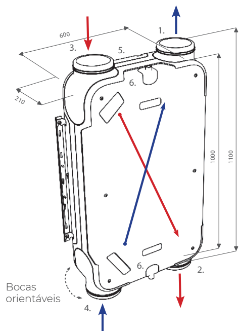
Fluxos de ar versão esquerda versão de fábrica Instalação horizontal no teto / vertical na parede
