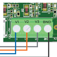
Regleta de conexionado de 3 velocidades en la PCB
