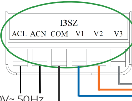
Regleta del mando
