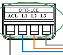
Regleta del mando
